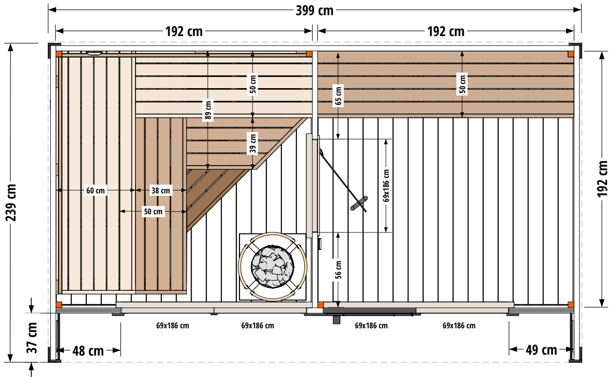
Draufsicht: Element Superb (Option L-Bank Dreistufig)
