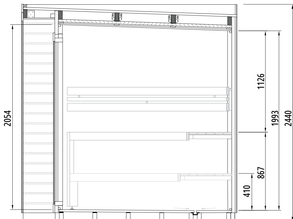
Querschnitt: Element Superb (Option Standardbank)
